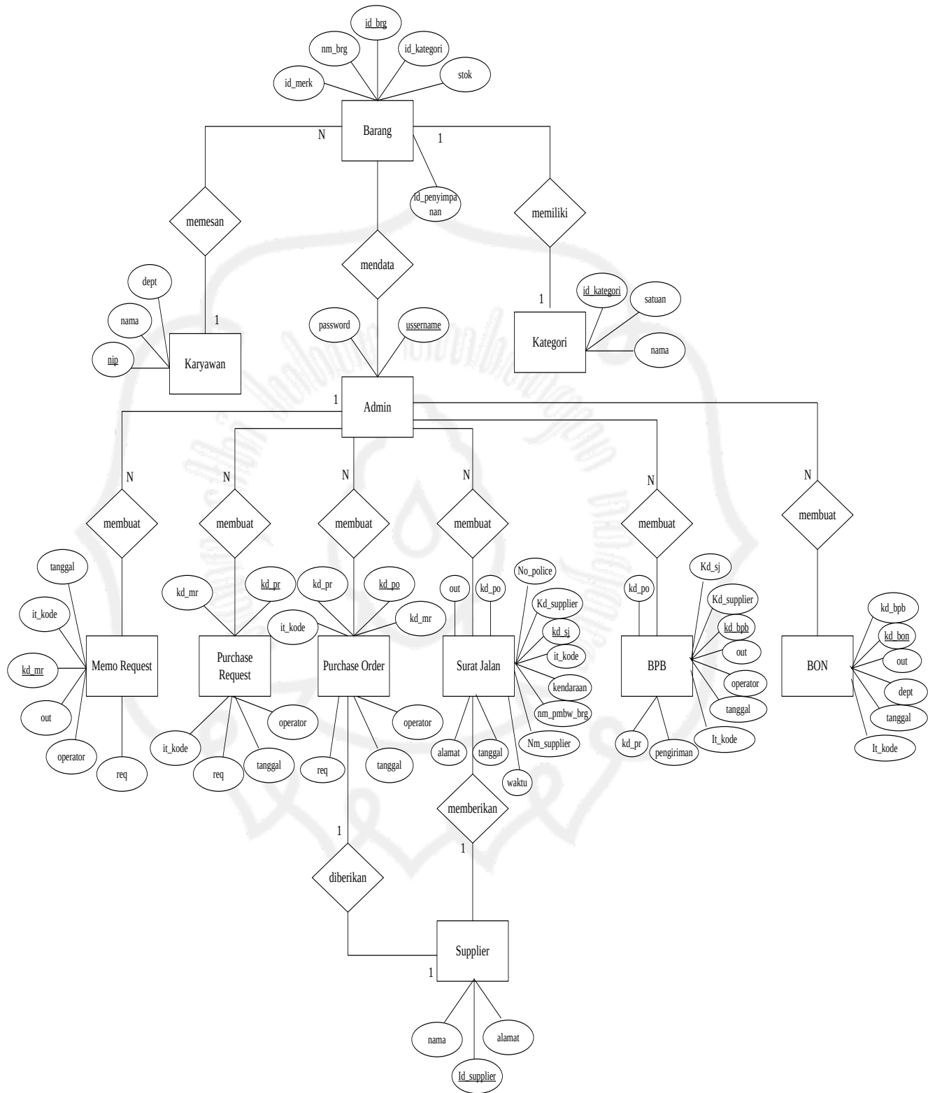
Gambar 14. ERD
